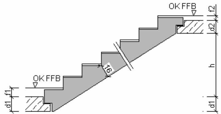
Doppelt gewendelte Treppe Typ 1 + 2 [m]
